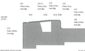
PRESTIGE EDGE DETAIL A1 SC 1/10 A3 SC 1/20
