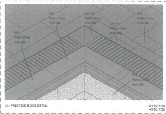
D1. PRESTIGE EDGE DETAIL
