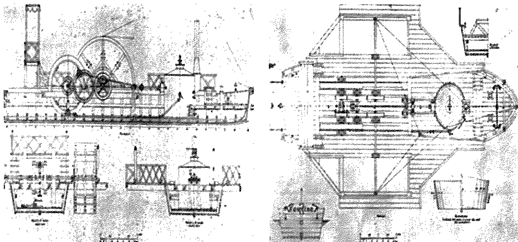
A CAROLINA rekonstrukciós rajzai. (Forrás: Várfalvy Tamás alkotása)
